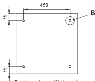
Zadní panel - montážní rozměry
