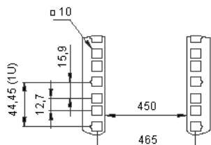
Montážní rozměry
