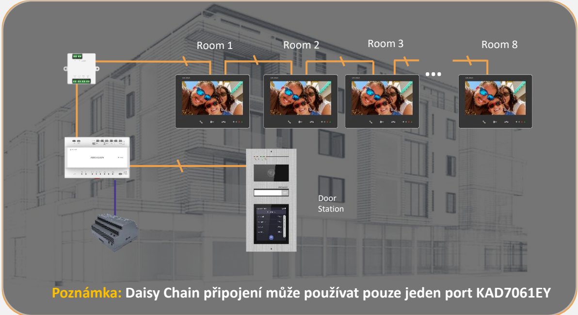
Zapojení řetězem přes DS-KAD7061EY (maximálně 8 vnitřních stanic)
