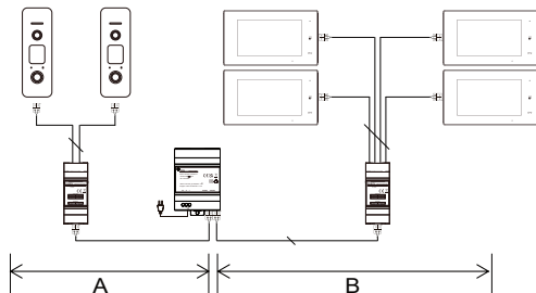
Strukturovaná kabeláž s rozbočovači s ochranou proti zkratu:
