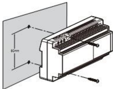
montáž šrobků na pevný podklad
